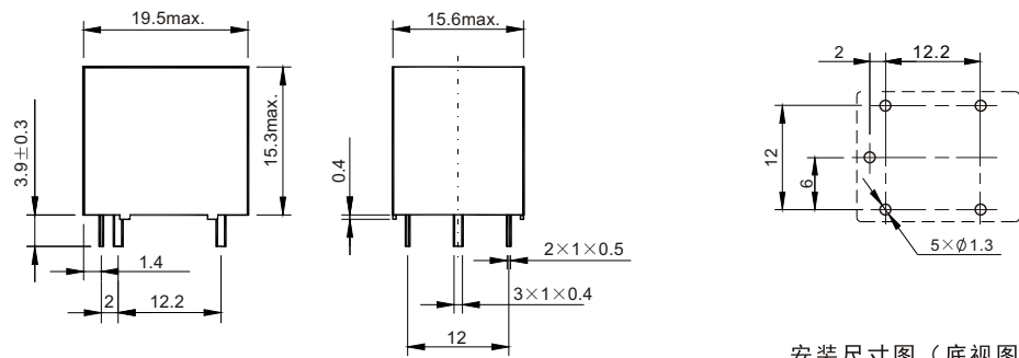
安装尺寸图 (底视图)
