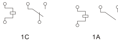
接线图 (底视图)
