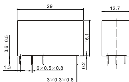
外形尺寸图
