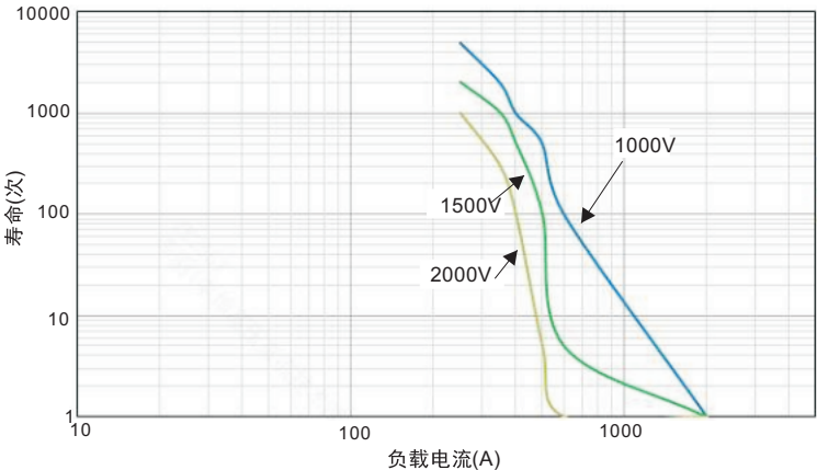
分断电寿命曲线
