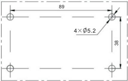
安装尺寸图
