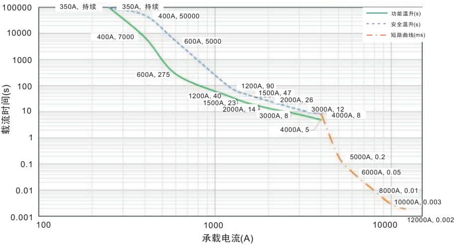
载流能力曲线
