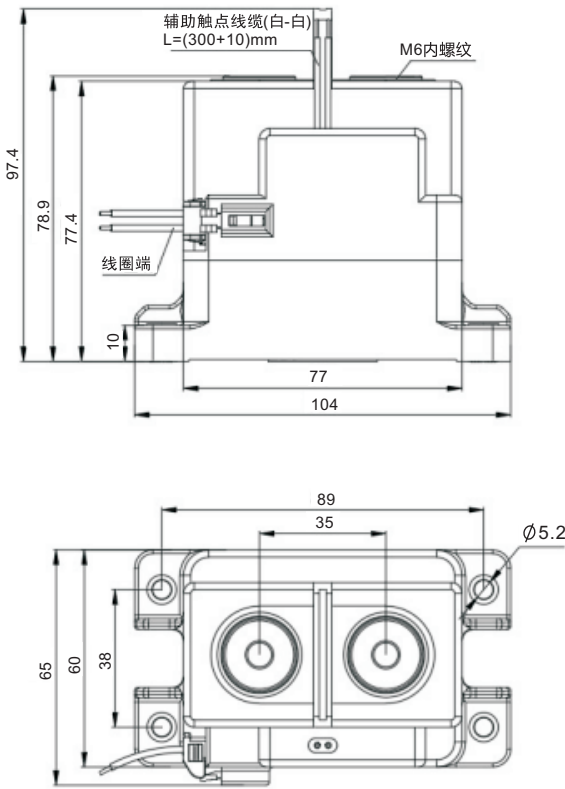
外形尺寸图
