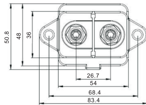
外形尺寸图
