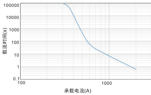
载流能力曲线
