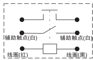
接线图
