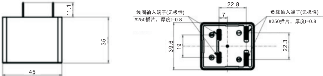
外形尺寸图
