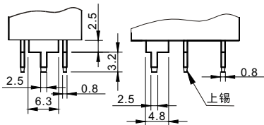
PCB式引出端
