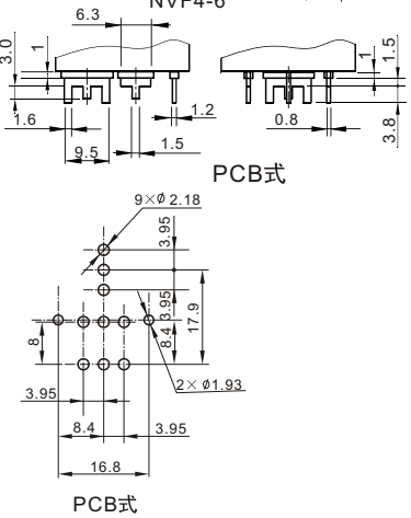
PCB式
