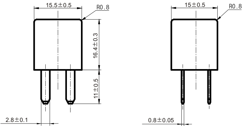
外形尺寸图
