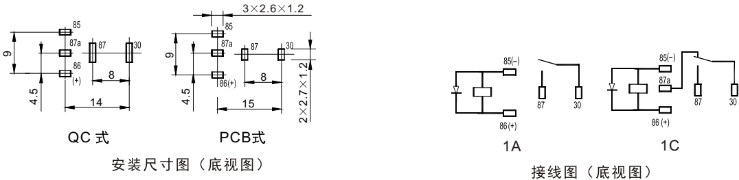
接线图（底视图）
