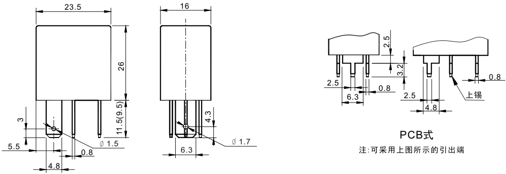
外形尺寸图
