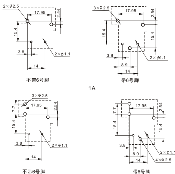
安装尺寸图（底视图）
