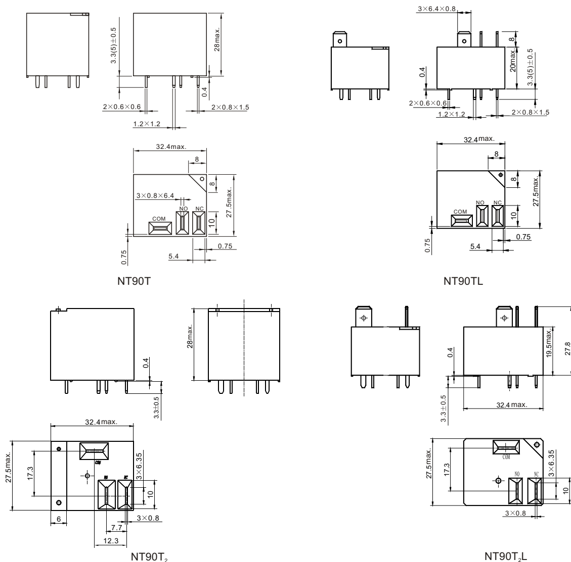
外形尺寸图
