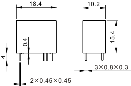
外形尺寸图
