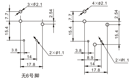
安装尺寸图（底视图）
