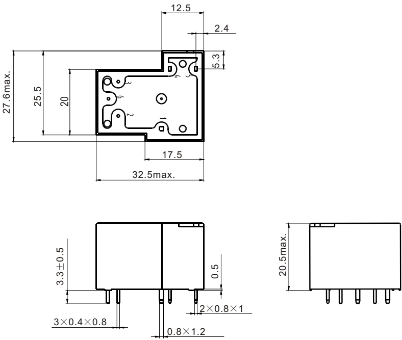
外形尺寸
