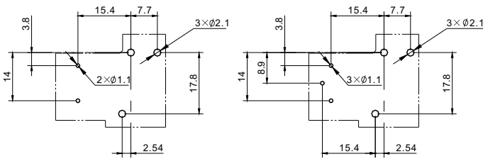
安装尺寸图（底视图） D 式
