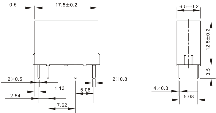
外形尺寸图
