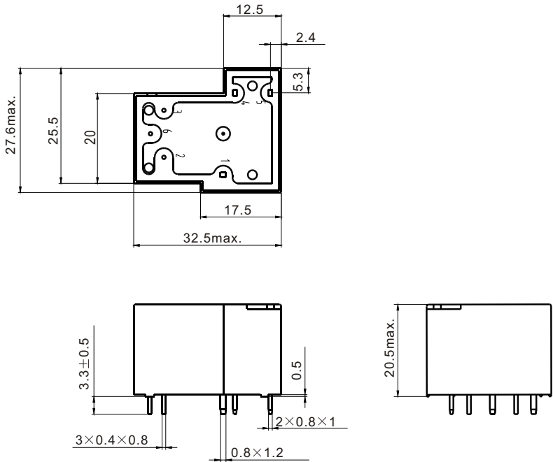
外形尺寸
