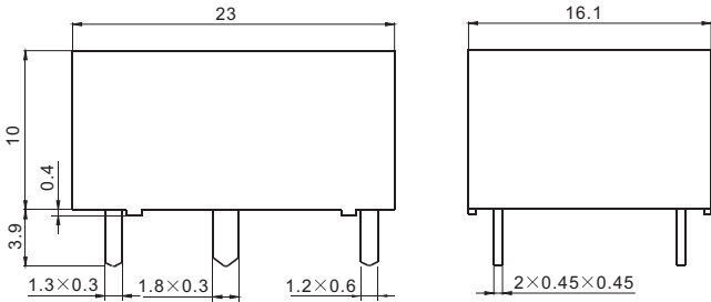
外形尺寸图
