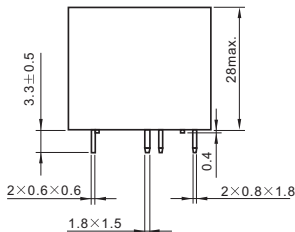
外形尺寸
