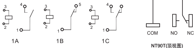
NT90T(顶视图)
