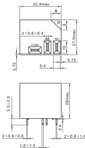
外形尺寸
