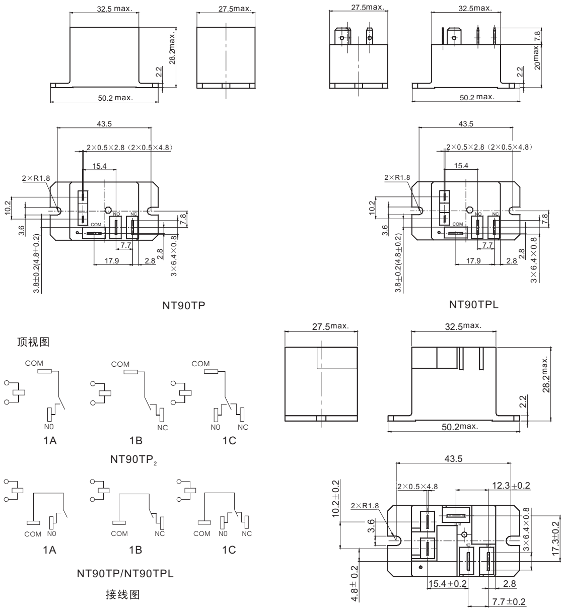
NT90TP 2 外形尺寸图
