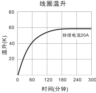
线圈温升
