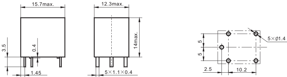
安装尺寸图（底视图）
