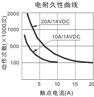
电耐久性曲线
