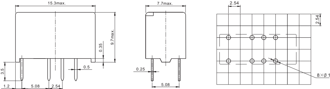
外形尺寸图
