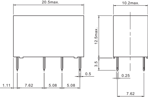
外形尺寸图
