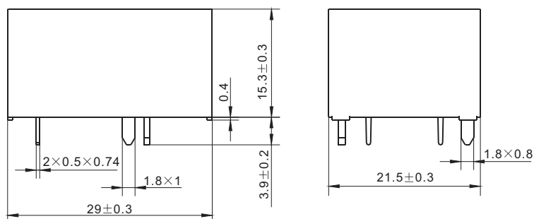
外形尺寸图
