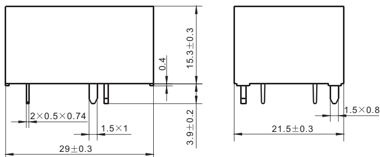
外形尺寸图
