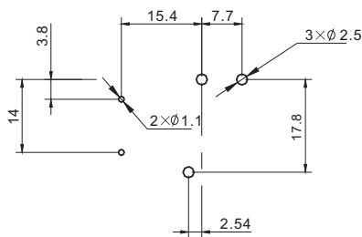
单线圈
