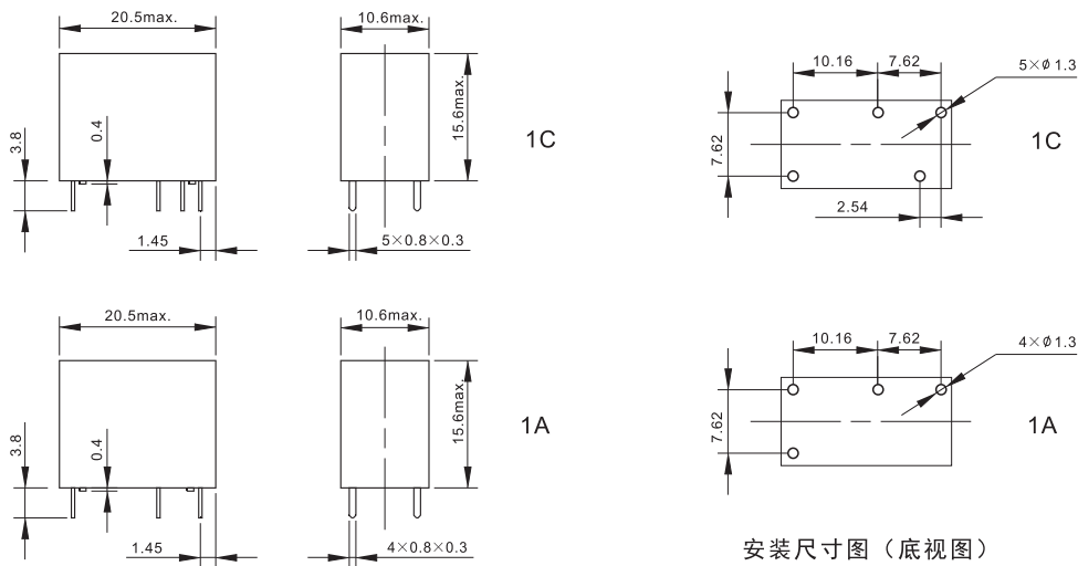
外形尺寸图
