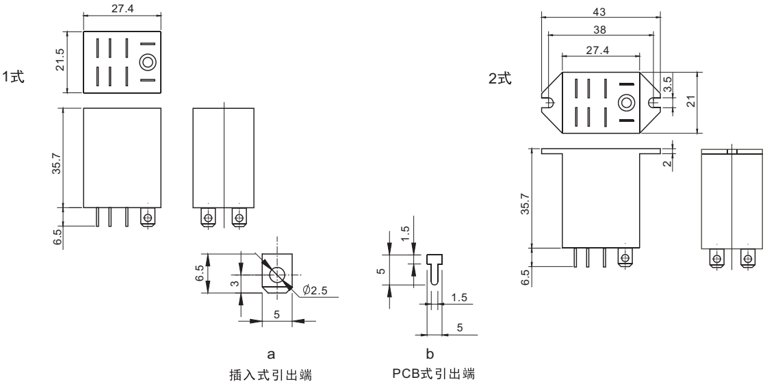
外形尺寸图
